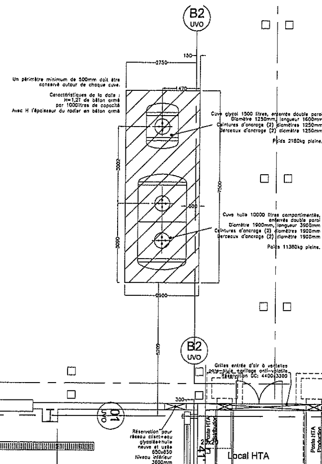
Implantation extérieure des cuves
