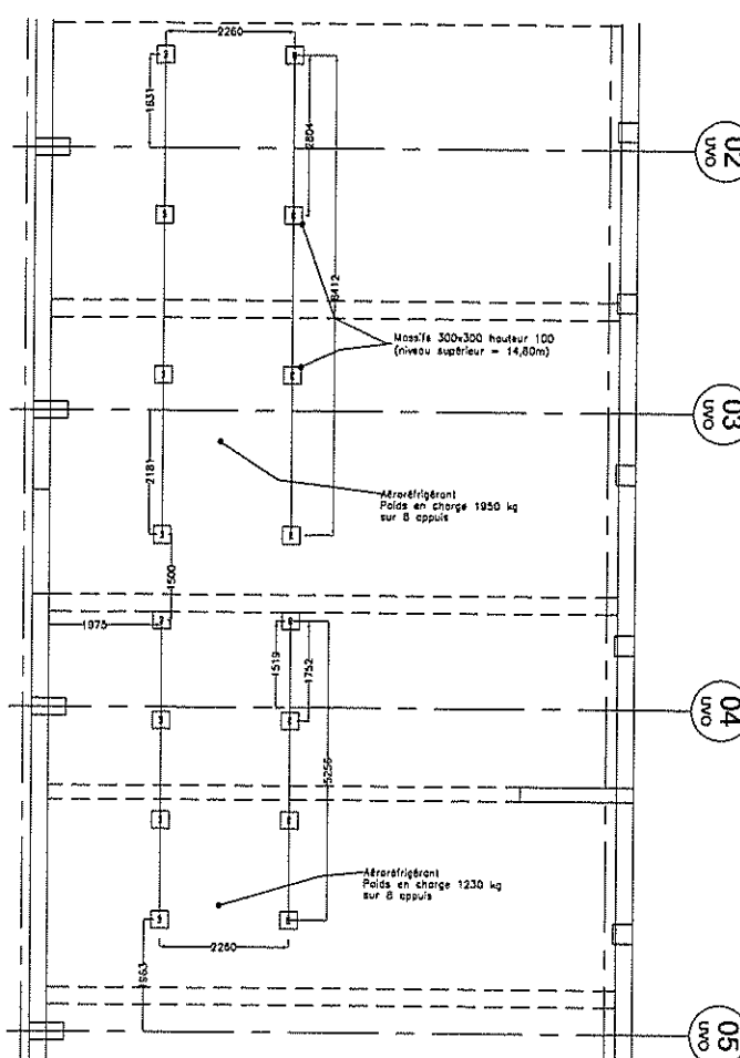
Vue en plan niveau +14.70m
