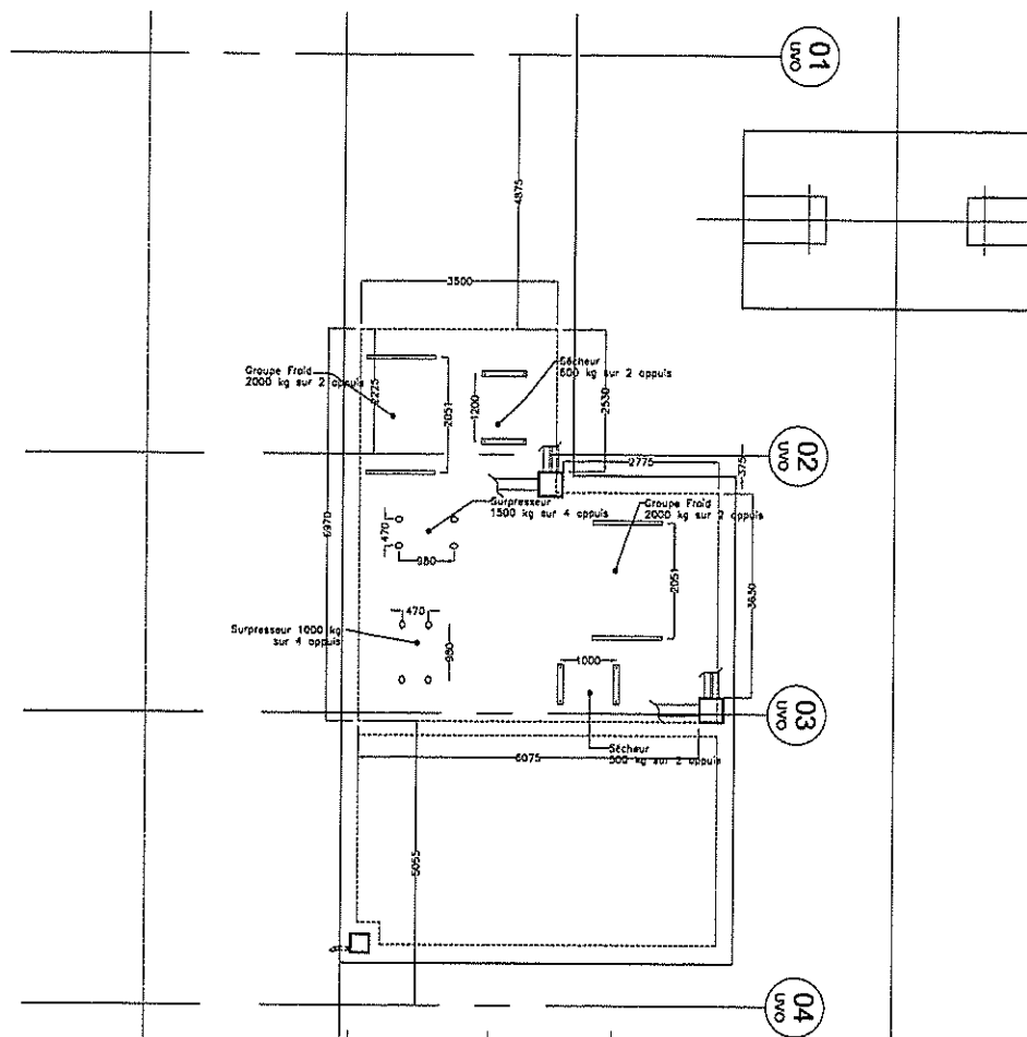
Dalle extérieure désulfuration
